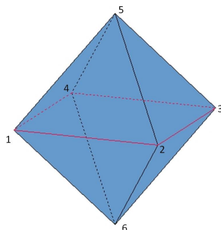
FIGURE 2 – Une réalisation du complexe de l'exemple 8. Le sous-complexe maximal de l'octaèdre engendré par les sommets 1,2,3 et 4 est le carré rouge.
