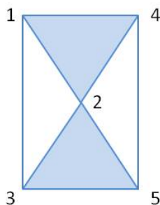
FIGURE 1 – Une réalisation du complexe de l'exemple 1
