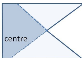
FIGURE 4 – Réalisation étoilée non convexe du pentagone. Le centre est l'ensemble des points de la zone plus foncé à l'intérieur de la réalisation du pentagone.
