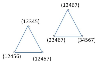
FIGURE 3 – Graphe d'un ensemble fondamental non minimal pour le PEUR
